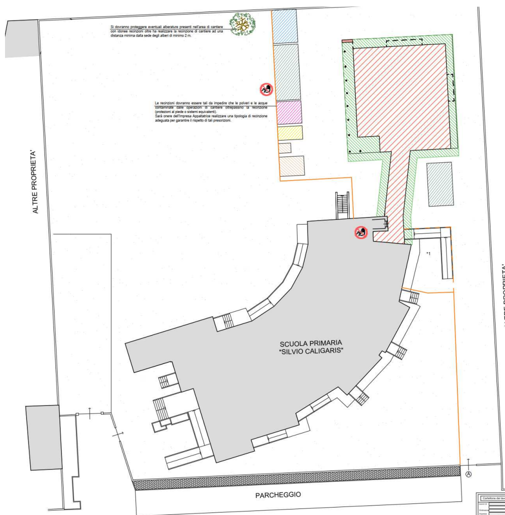
Figura 2 – Layout di cantiere
